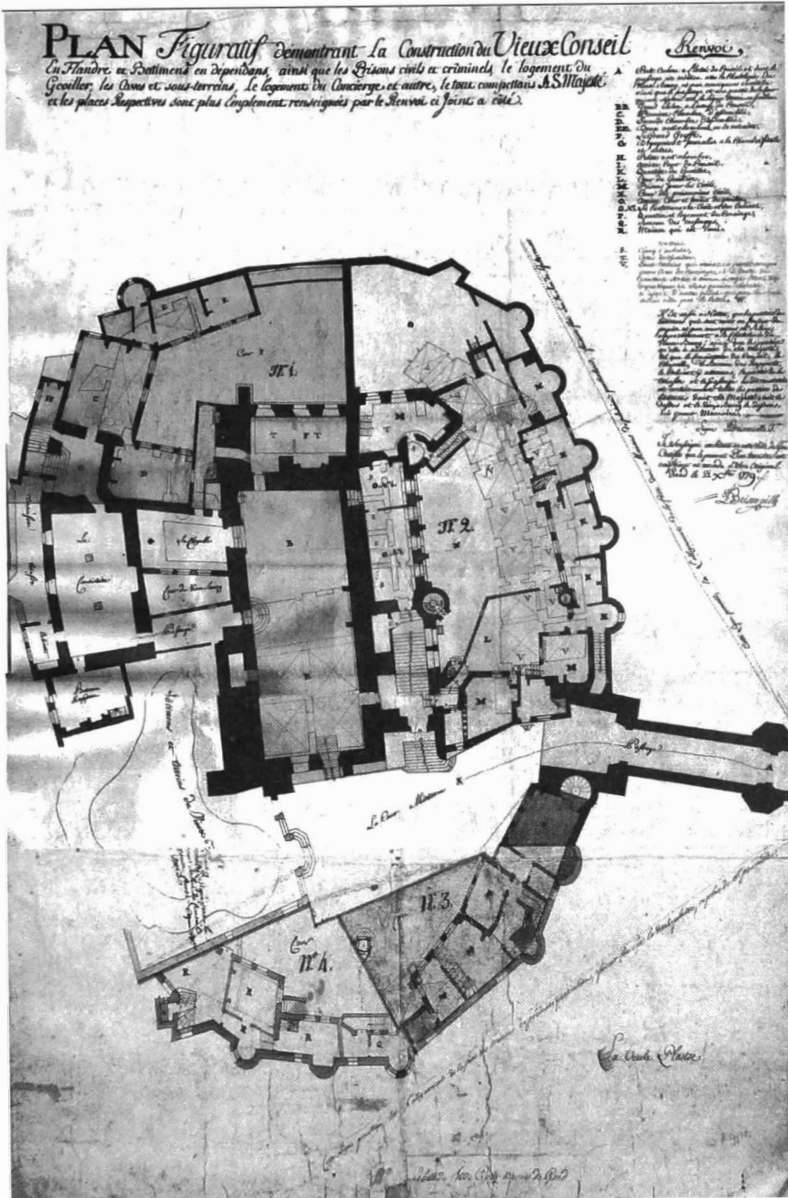
Afb. 2. Plattegrond van het Gravensteen in 1779 door Jean-Denis Brismaille - kopie (Stad Gent, De Zwarte Doos, Stadsarchief, Atlas Goetghebuer, lade 40 nr. 8).
