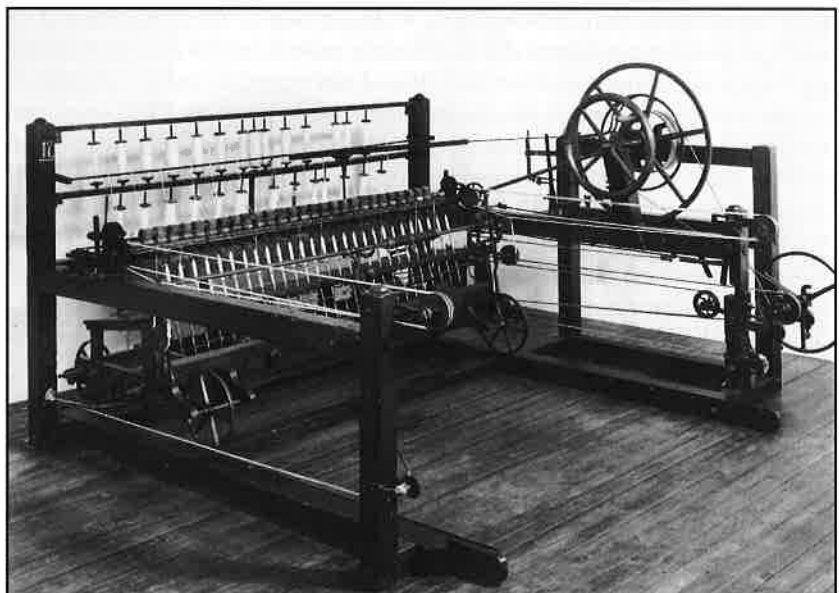
De 'mule jenny' in het MIAT. De spinmachine die circa 1800 door Lieven Bauwens in Vlaanderen werd geïntroduceerd. (foto Claerhout Gent, verzameling MIAT)
