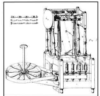
'Waterframe' (uit: De Mule Jenny , 1982, MIAT)
