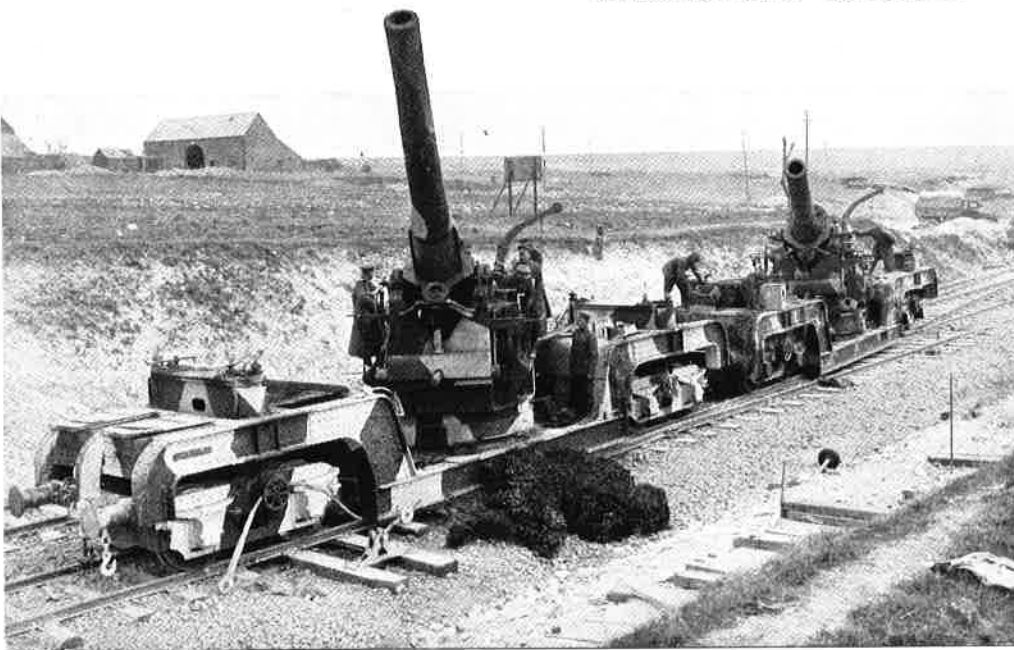
Zwei erbeutete englische Langrohrgeschütze auf einem Schienenstrang im Kampfgebiet vor Péronne
