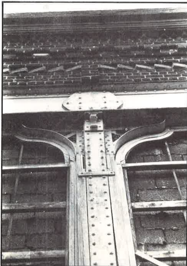
detail metaalpijler raamconstructie spinnerij
