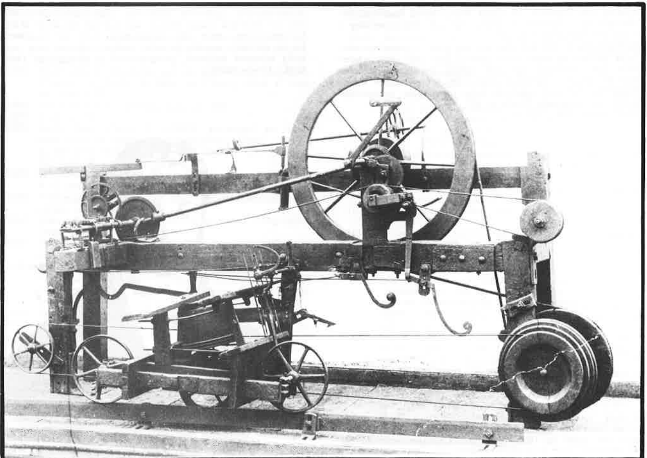
Enig behouden fragment van de originele Spinning Mule van Samuel Crompton, waarbij het halfautomatisch aandrijfmechanisme en de uitloopwagen duidelijk zichtbaar bleven (Lewis Textile museum, Blackburn). (Foto Archief M.I.A.T., Gent)
