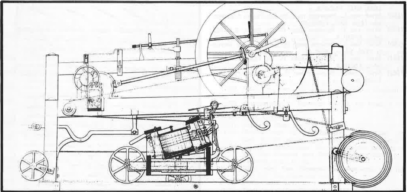
Opmetingstekening van originele Spinning Mule , ontwikkeld door Samuel Crompton te Bolton tussen 1779 en 1780. De basisstructuur zoals ook aanwezig in de Gentse mule jenny , is duidelijk herkenbaar (aandrijf wiel, overbrengingsstang, wagen, uitrekbank). (Foto Archief M.I.A.T., Gent)
