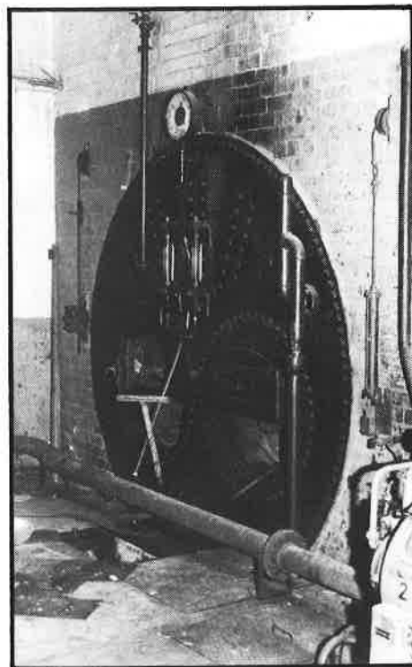
Stoomketel "P. Brouhon, médailles d'or : Amsterdam 1883 - Anvers 1885. Pierre Brouhon, Liège - diplôme d'honneur Anvers 1883" geplaatst in de spinnerij De Smet-Guequier.
