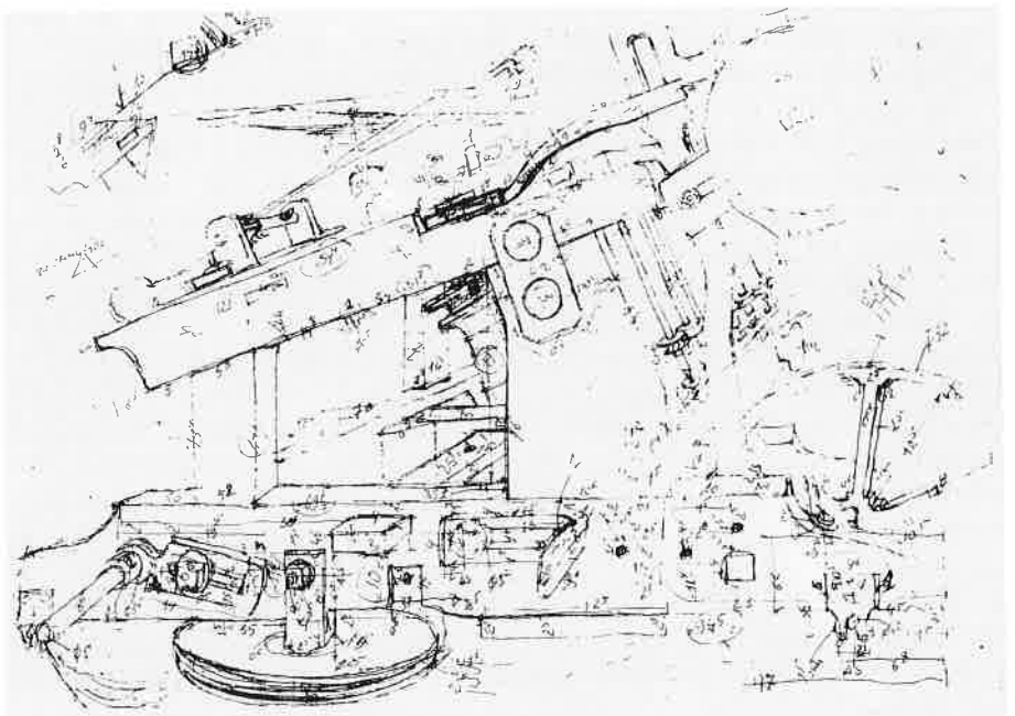
Opmetingsschets van de mule jenny, uitgevoerd in het kader van het OPVIT
