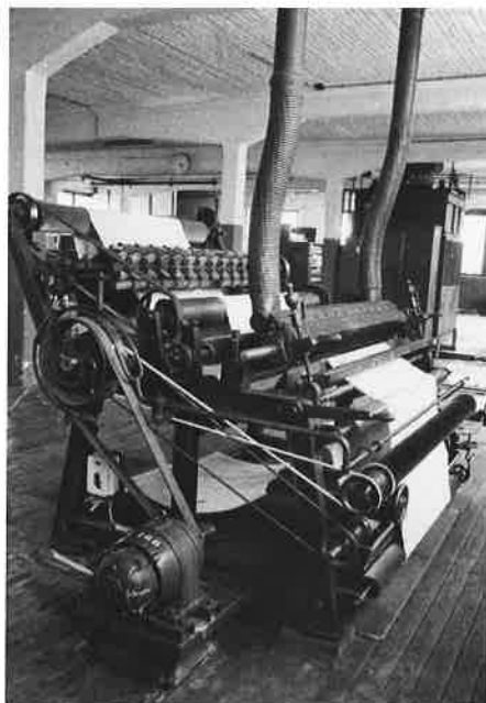
Mechanisch Jacquard weefgetouw, regionaal fabriekaat 'Ateliers. Vve Mathieu Snoeck te Eusival, ca. 1930) (links)
