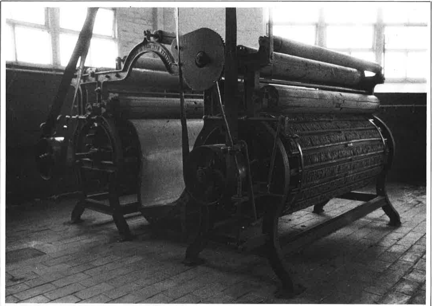
Ruwmachine voor wollen lakens, vervaardigd in het Vervierse constructieatelier G.G. Bosson (1914)
