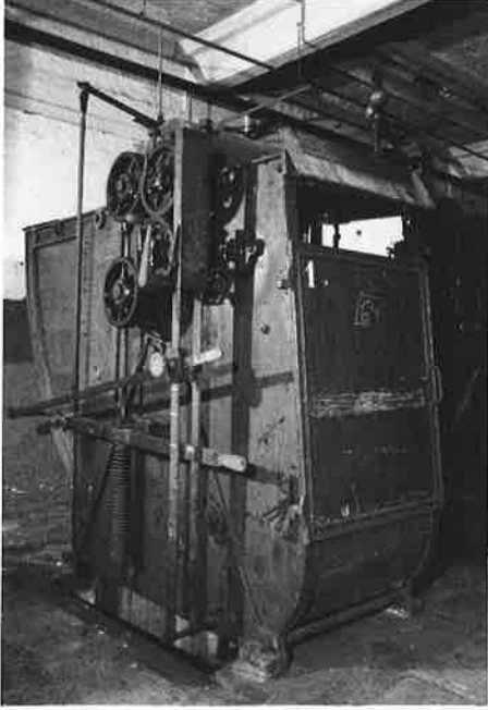
Volmachine, regionaal fabricaat (Ateliers Raschon, ca. 1950)
