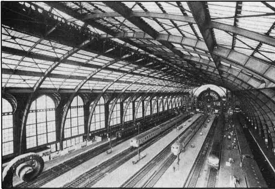
Het Centraal Station van Antwerpen. De reusachtige metalen overkoepeling van dit derde station op deze plaats, werd in zijn huidige vorm opgetrokken in 1895-1899 n.o.v. architect Louis de la Censerie. De monumentale voorbouw dateert uit 1900-1905. (uit: P. VIAENE en R. DE HERDT, Industriële Archeologie in België , 1987, MIAT, Gent).
