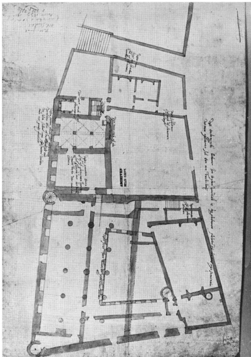
3. Grondplan van een deel van de oude seminariegebouwen. Opgemaakt door de architect Jacques Francquart in 1626 met het oog op de verbouwing tot een tuchthuis; toen waren aan de gebouwen sinds het begin van de 16e eeuw belangrijke veranderingen aangebracht. Onderaan, langs de Schelde, rechts het Gerard Duivelsteen waarin de kapel van de Fraters en van het Seminarie was gevestigd; links daarvan blijkbaar de klaslokalen en de toiletten (goederenlijst, nr 5). Uiterst links boven het gebouw nr 6. Boven rechts, aan de Nederscheldestraat, de refter van de studenten (nr 3). Tussen dit laatste en het Gerard Duivelsteen een kloosterpand, gebouwd door de Fraters. Het complex strekte zich verder uit naar het noorden (rechts) tot op de Wijdenaard, het huidige Bisdomplein (Gent, Stadsarchief).
