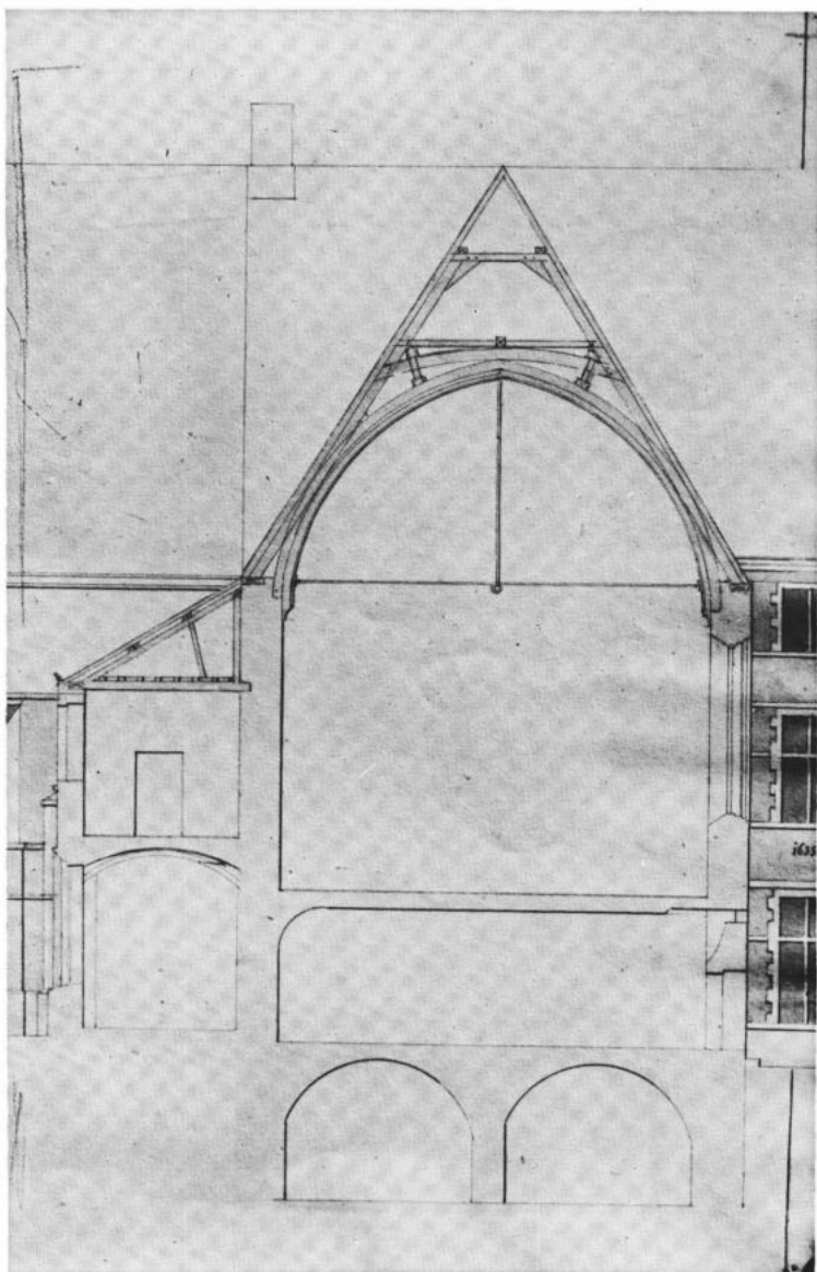
Afb. 25 — Refter, kruisgang, korte doorsnede.
