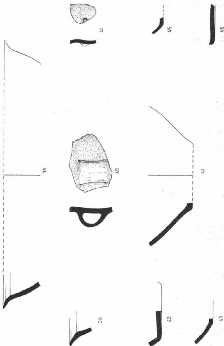
Fig. 10. KW 1,6. IJzertijdardewerk. Schaal \frac{1}{3} .
