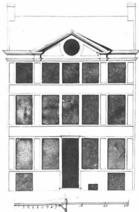
11. Gevelontwerp voor de herberg "De Cleyne Sterre", bij het belfort, 1778 (SAG, 535, 282/18).
