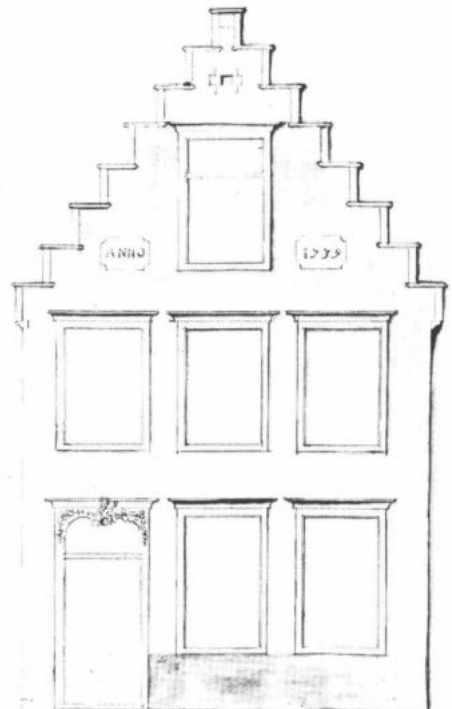
5. Gevelontwerp voor de herberg "Den Bacchus", bij de Oordeelbrug, 1739 (SAG, 535, 215/1).
