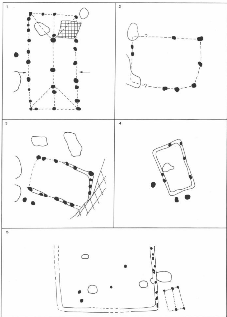
Fig. 6. Detailplan van de gebouwen van Huise-Lozerbos (1-4) en van Vinderhoute-Molenbrug (5). Schaal 1/150.
