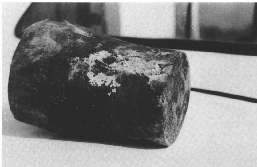
Bij een Turkse vuurmond uit circa 1476, opgevist uit de zee vóór Noord-Israël, vond R. ROTH de houten plug nog op de kruitkamer steken. Haifa Maritiem Museum. Foto R. ROTH.
