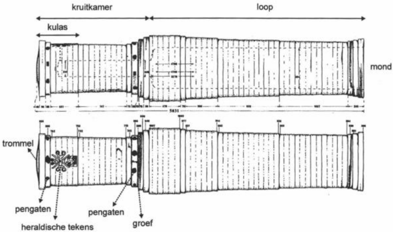
Structuurschets van de buitenzijde van de Dulle Griet door R. ROTH, Schwarzenburg, oktober 1998.
