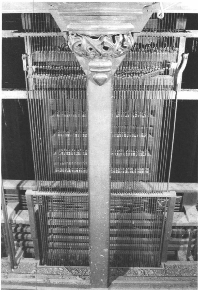
Afbeelding 3 Barkermachine frontaal
