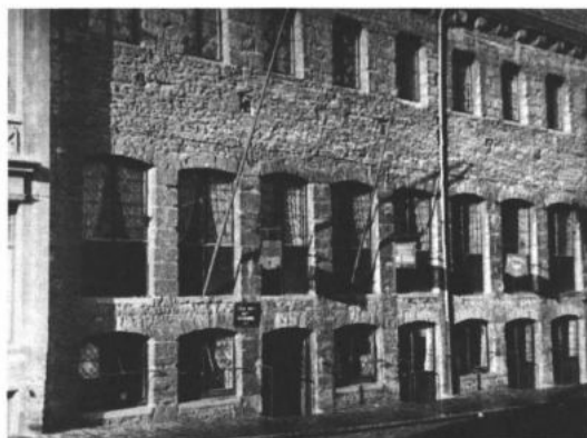
Afbeelding 4 Op de begane grond hebben de doorbrekingen een segment-boogvormige afdekking die wordt herhaald op de eerste verdieping. Tijdens de restauratiewerken in 1904 stelde architect Ernest Van Hamme vast dat de doorbrekingen op de eerste verdieping, die tot dan toe als vensters waren ingevuld, in oorsprong deuropeningen waren (SAG., Reeks SCMS, Foto's, doos 165, Hooiaard, nr. 2390)
