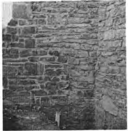
Afb. 23 — Centrale steunbeer van de O.L.V.-kapel - detail metselwerk
