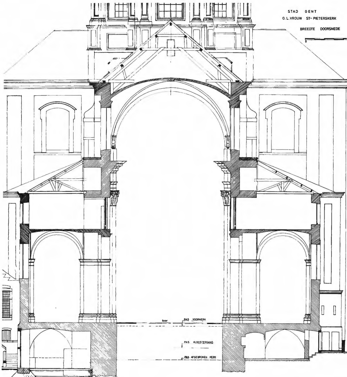
Afb. 11 — Breedtedoorsnede over het koor van de barokkerk volgens opmetingen van Arch. Dr. R. van Driessche
