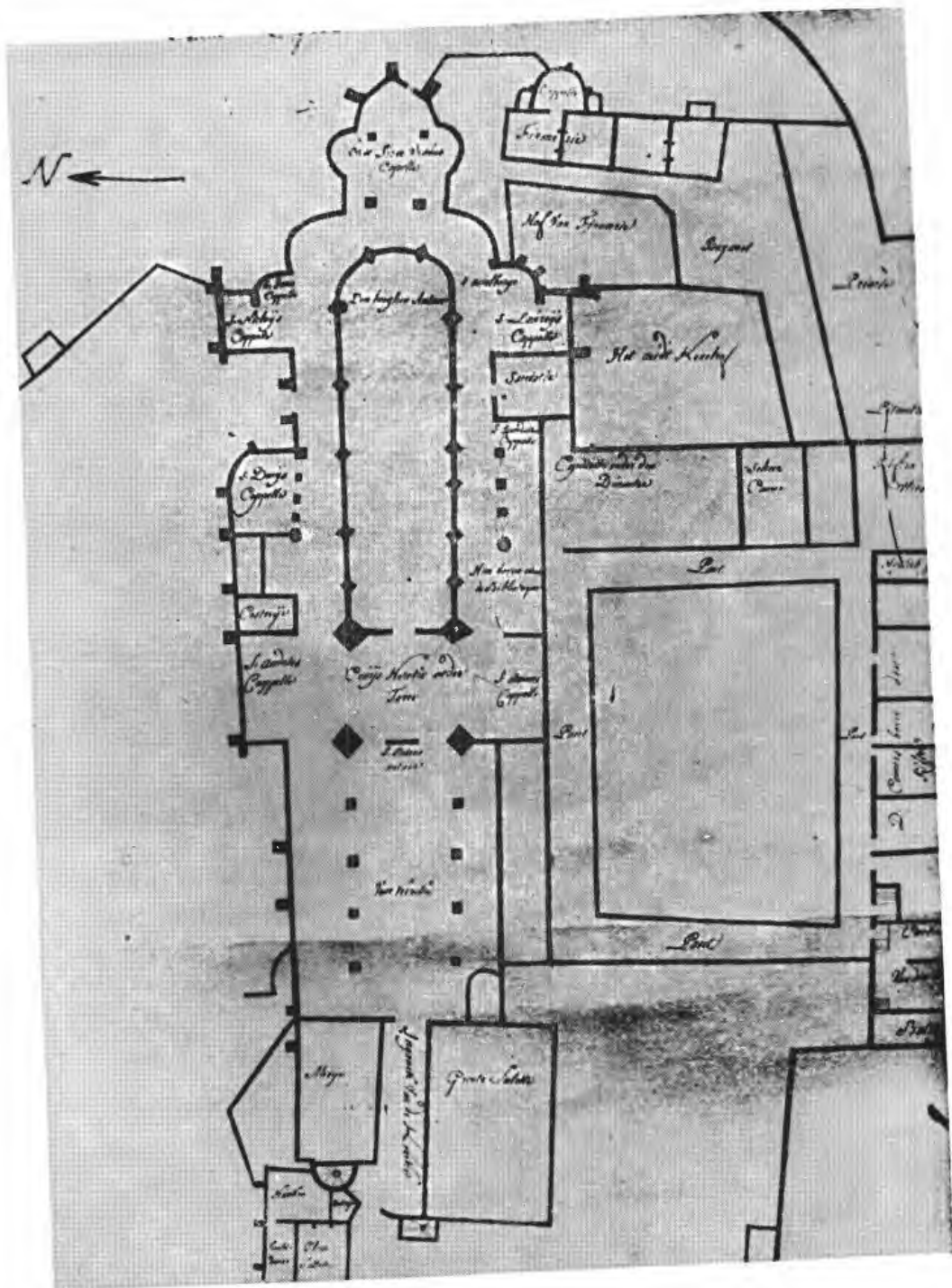
Afb. 6 — Detail van het „Rode Plan”, Rijksarchief, kaarten en plans, nr. 205. Voor Afb. 7 — zie blz. 16-17 van de tekst
