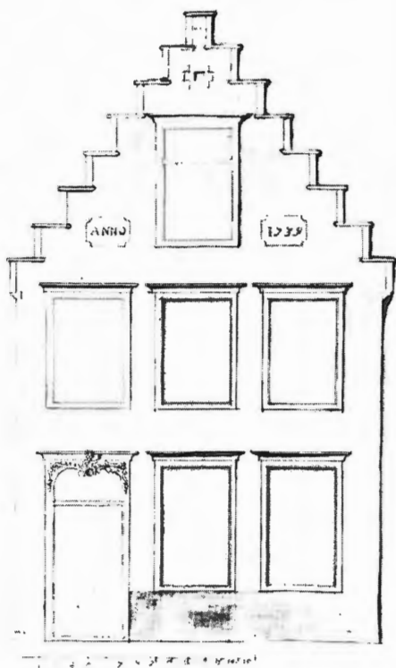
5. Gevelontwerp voor de herberg "Den Bacchus", bij de Oordeelbrug, 1739 (SAG, 535, 215/1).
