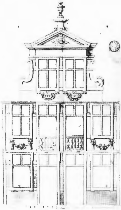
6. Gevelontwerp voor de herberg "Den Druyftack", Steendam, 1708 (SAG, 535, 310/6).
