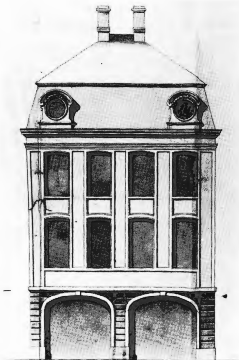
12. en 13. Ontwerpen voor de voor- en de achtergevel van de herberg "Het Oragne Boomken", bij de Walpoortbrug, 1771 (SAF, 535, 344/10).
