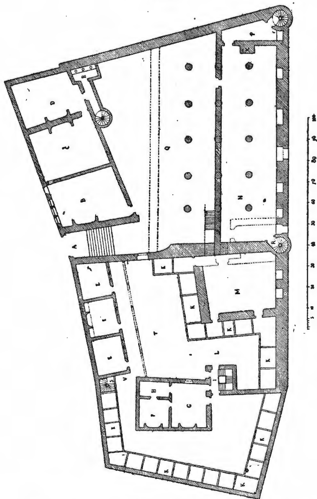
Le Château de Gérard le Diable à Gand, aménagé en Rasphuys en 1626(7) par l'ingénieur-architecte J. Francquart. Sous la lettre K sont indiquées 28 cellules de nuit.
