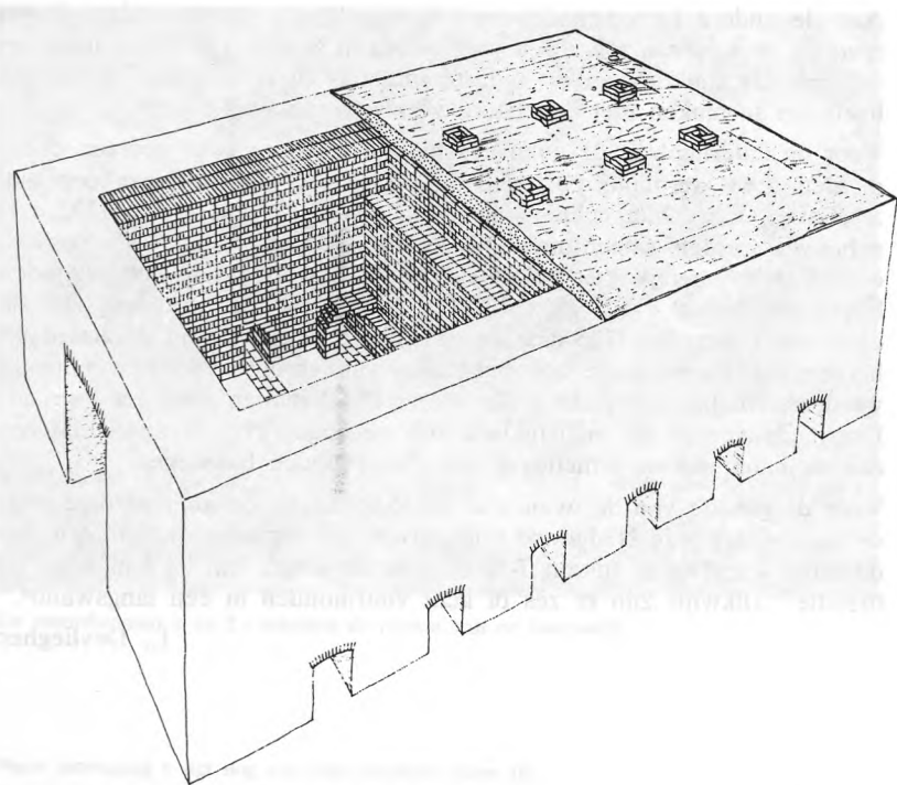
Reconstructie van een veldoven met zes vuurmonden.
