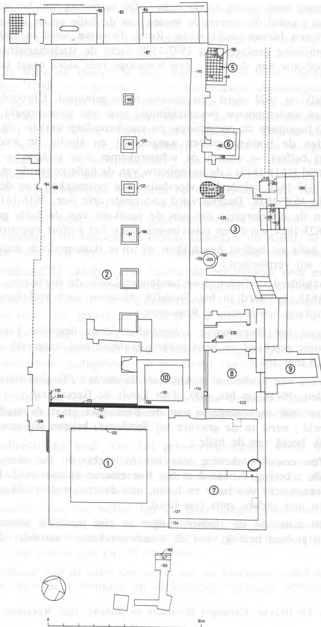
Grondplan van de funderingen van de halle en het belfort.
