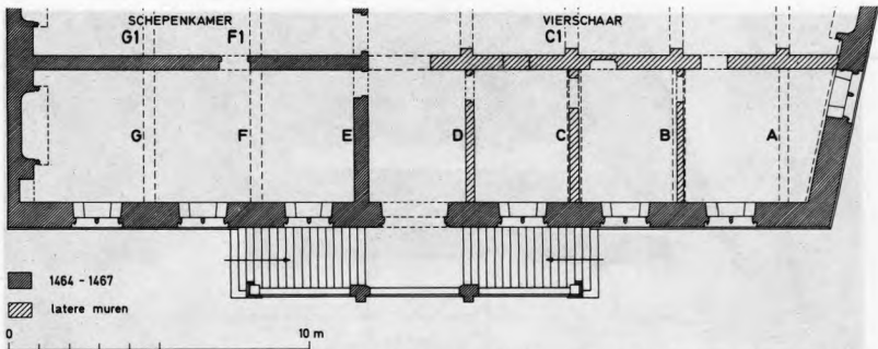
Damme, stadhuis. Gedeeltelijk grondplan van de bovenverdieping, met aanduiding van de moerbalken A-G.
