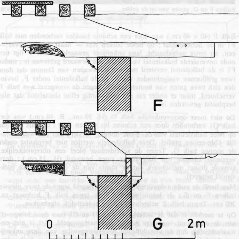
Moerbalken F en G en — links, in de Schepenkamer — F1 en G1.
