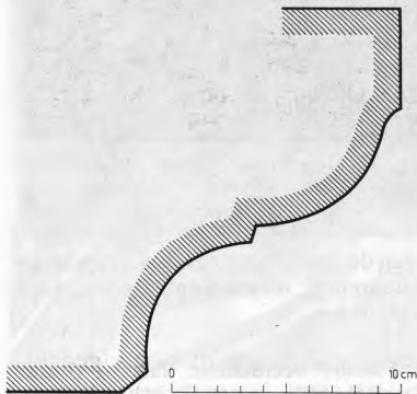
Profiel van een 17de-eeuwse blauwstenen konsole.
