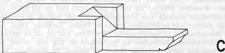
De verbinding van de 15de-eeuwse moerbalk C1 met de 17de-eeuwse balk C.
