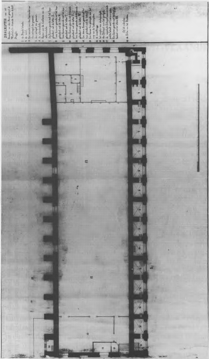
«Description van het bovenplan van den Bauw geseijt de Waterhalle». Anoniem, kopie uit de 19e eeuw (Rijksarchief Brugge).
