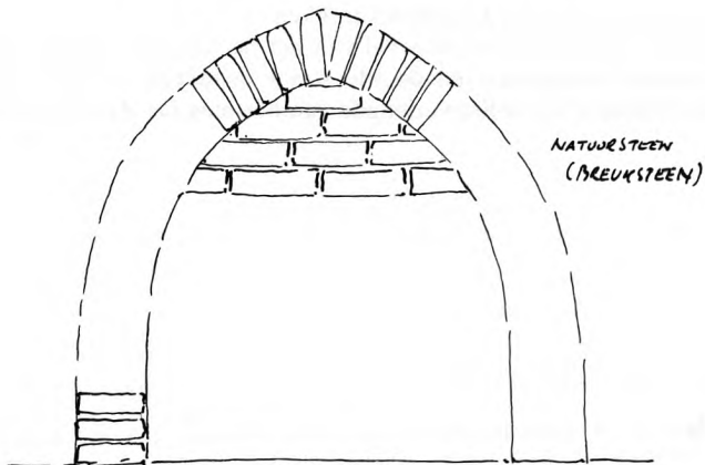
Schouw in de kelder van het ambachtshuis van de Schoenmakers.
