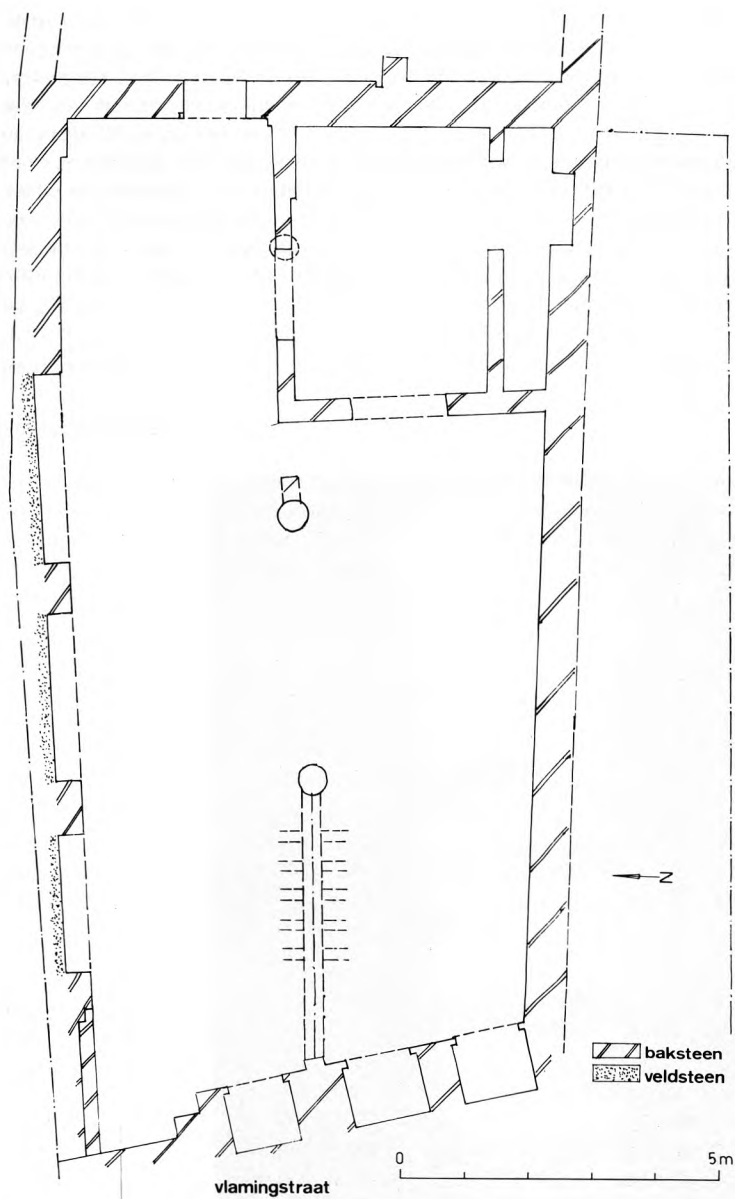
Grondplan van de kelder.
