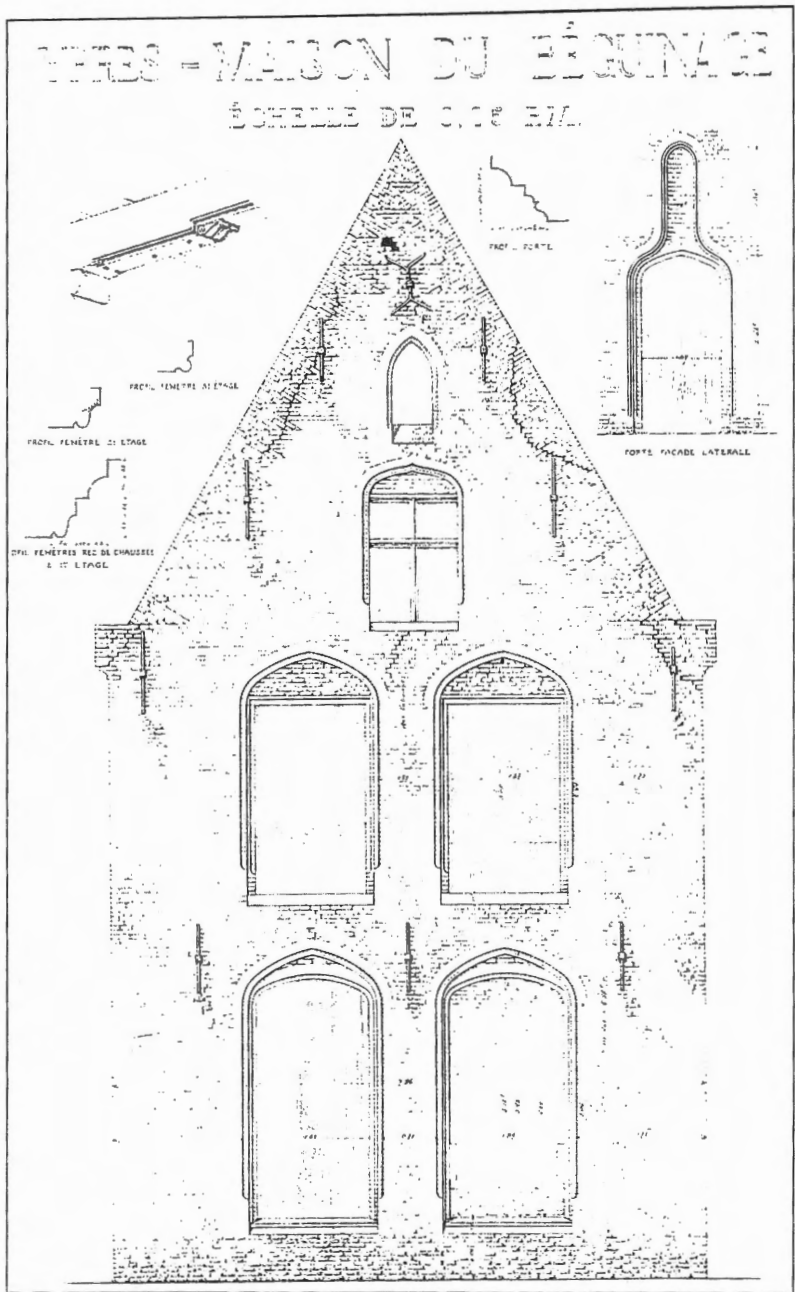
Tekening van een huis in het begijnhof in 1917. (uit H. Stynen e.a., Het verwoeste gewest. 15/18 Mission Dbnicque , Brugge, 1985)
