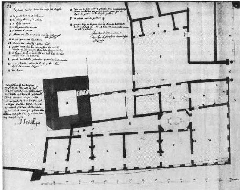
Plan II van architect J. Verkrus, goedgekeurd op 24 mei 1721, voor de nieuwe gebouwen van het Brugse Vrije. N.: "den toorn". (Brugge, Rijksarchief, Kaarten en Plannen, nr. 255/1).
