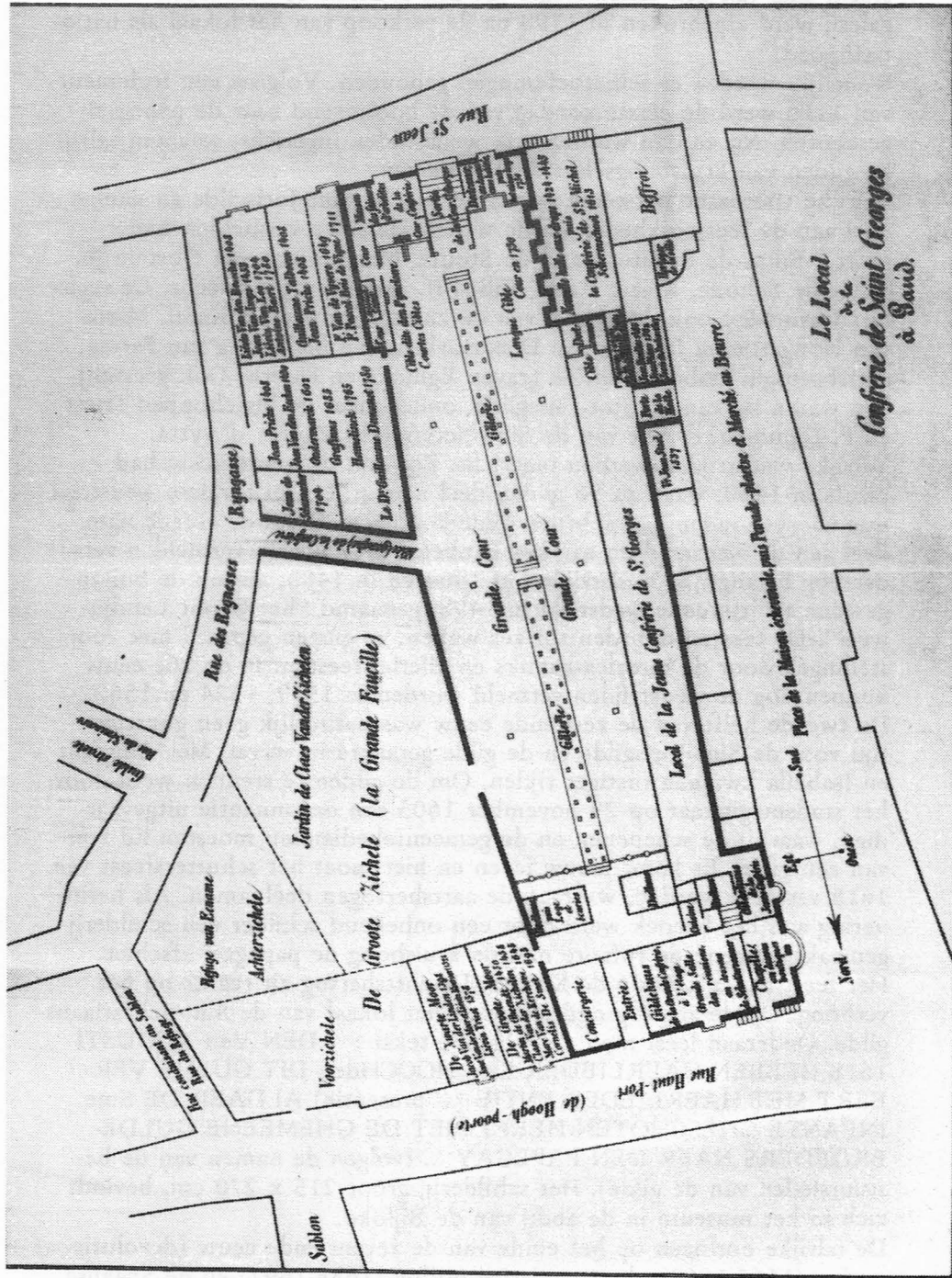
Plan van het Sint-Jorishof
