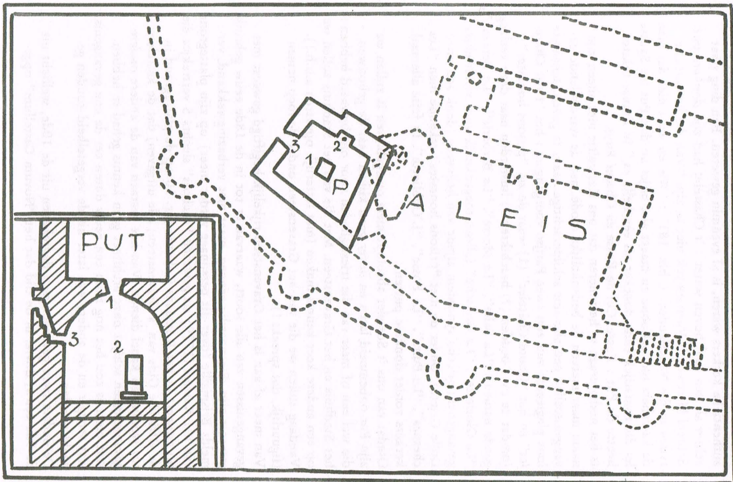
Plattegrond van Paleis met ligging van de Put; doorsnede van de Put op schaal van 1/200 naar tekening van A. van Werveke; 1 = gat; 2 = privaat; 3 = luchtkoker
