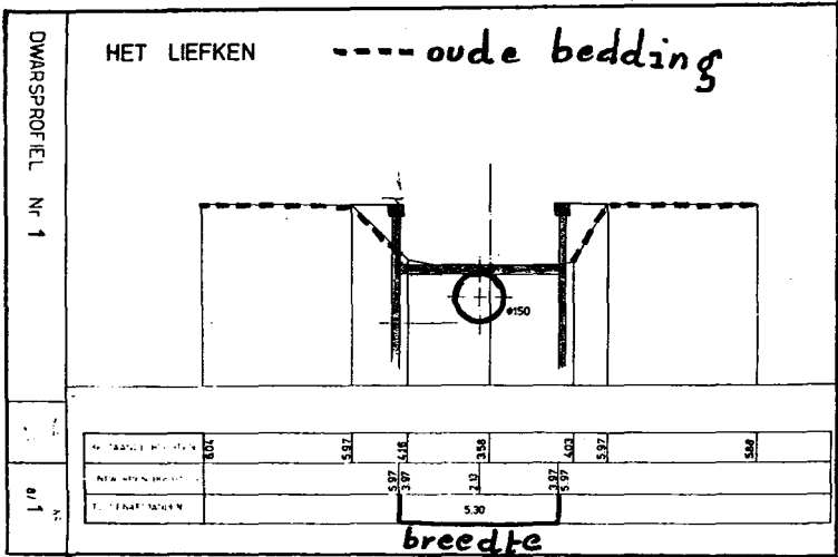
Fig. 2. Oud en nieuw dwarsprofiel van de Lieve
