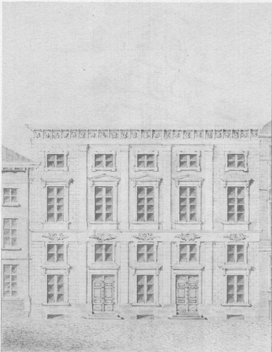
Sodaliteit omstreeks 1840.
