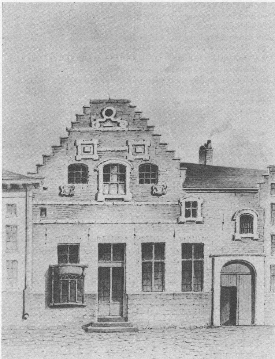
Sodaliteit omstreeks 1820.
