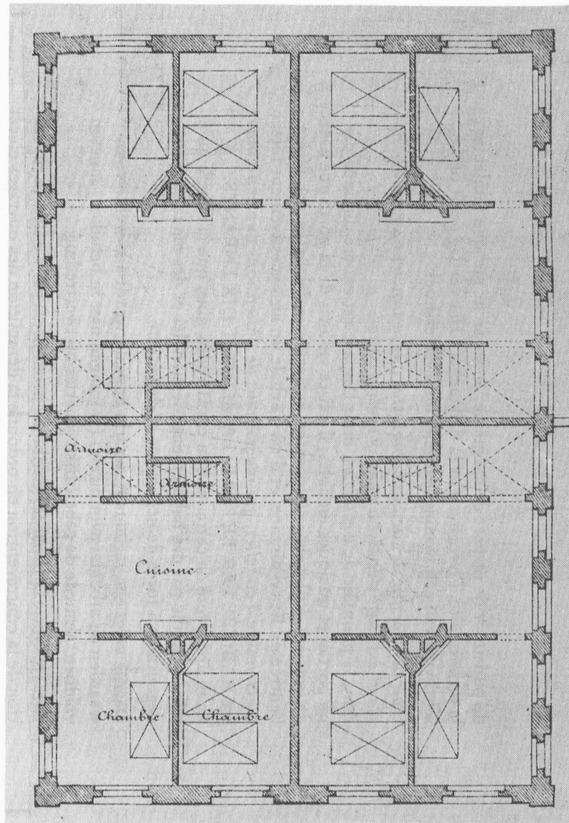
Plan van een arbeiderswoning. Elk gebouw omvat twaalf woningen. Elke woning is 7,5 m op 6 m. en bestaat uit een keuken van 6 m op 3,75 m en twee slaapkamers van 3 m op 3,75 m. Naast elk gebouw ligt een tuintje.
